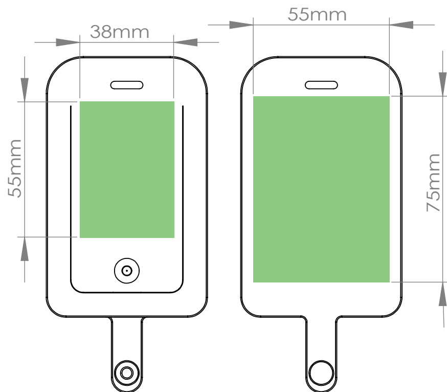
網版印刷
